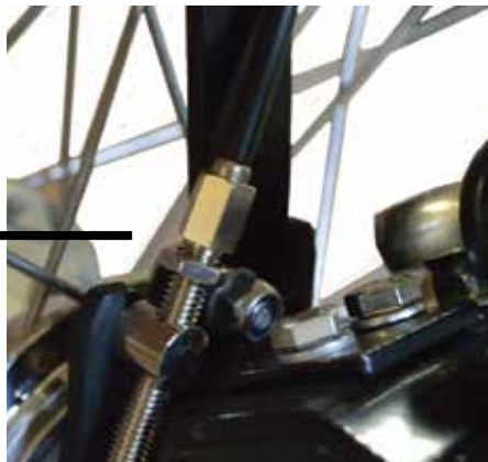
Justering af håndbremsekablet
